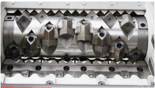
单轴刀具
